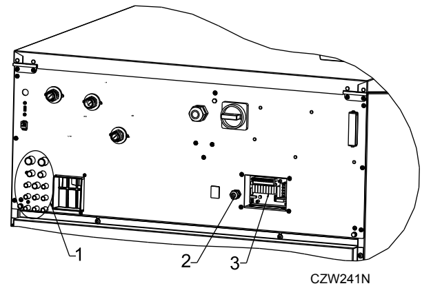
Panneau de valve – Vue arrière
